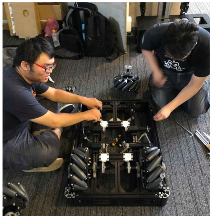
本團隊隊伍成員進行機器人硬體組裝
